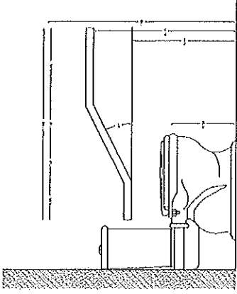
ALZADO LATERAL BARRA NIÑO DISCAPACITADO
